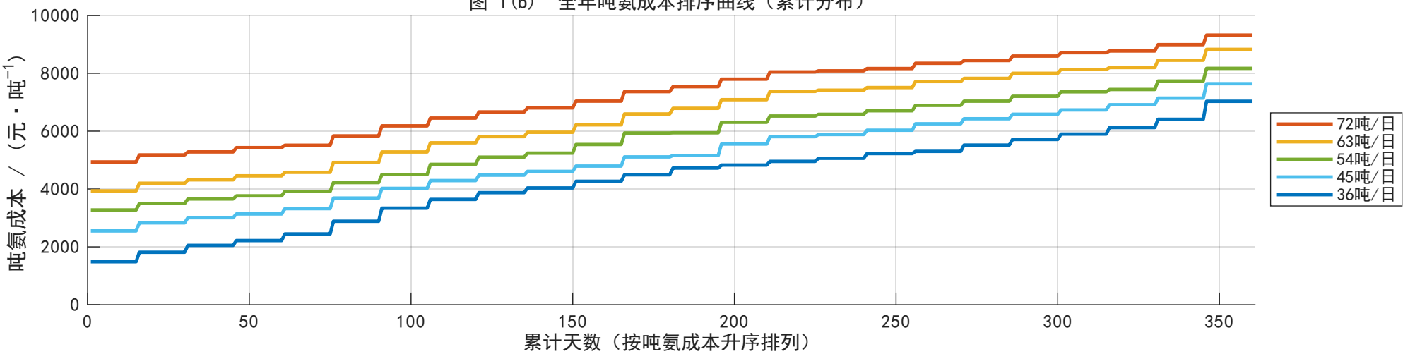
图 1(b) 全年吨氨成本排序曲线（累计分布）
