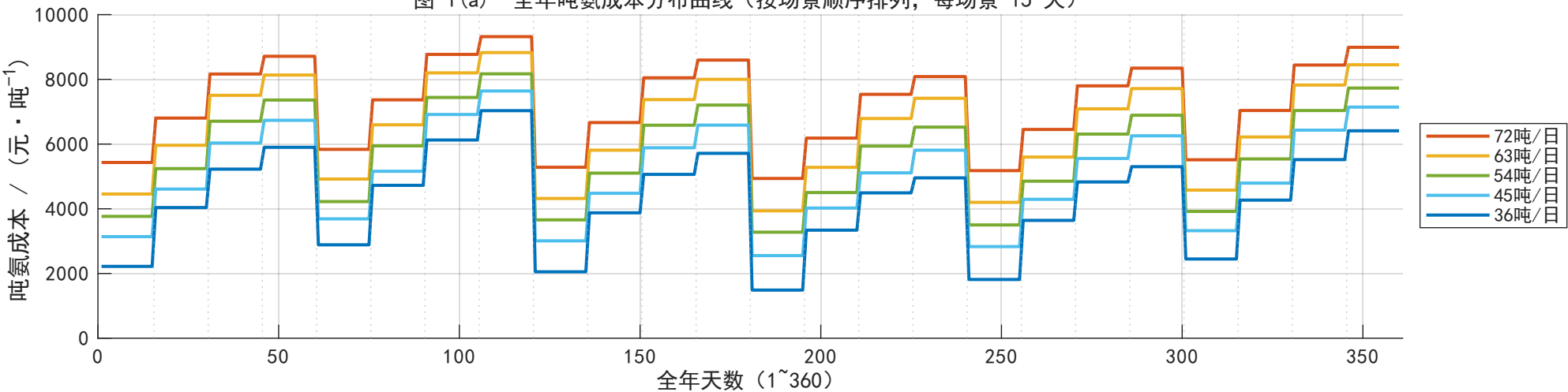
图 1(a) 全年吨氨成本分布曲线（按场景顺序排列，每场景 15 天）
